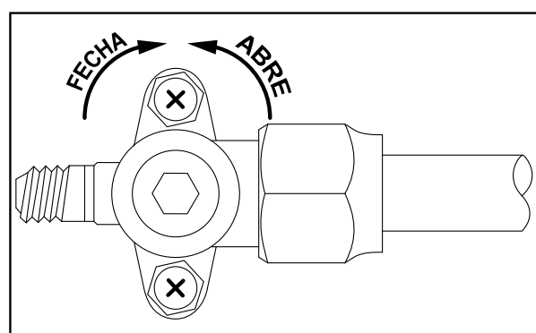
FIG. 19 - VÁLVULA DE SERVIÇO SEM PORCA DE PROTEÇÃO
