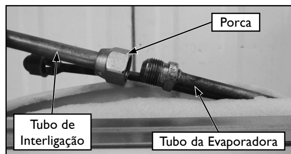
FIG. 27 - CONEXÃO DA LINHA DE SUCCÃO
