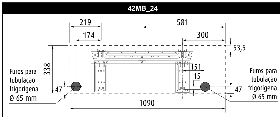
FIG. 14-B - PLACAS DE MONTAGEM
