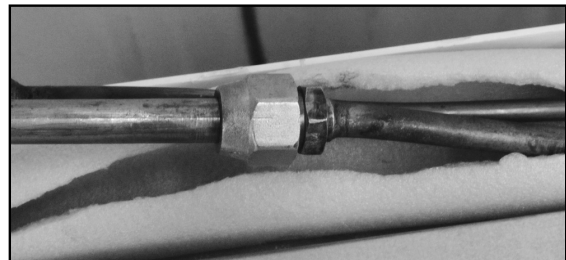
FIG. 28 - CONEXÃO DA LINHA DE SUCCÃO DA UNIDADE EVAPORADORA
