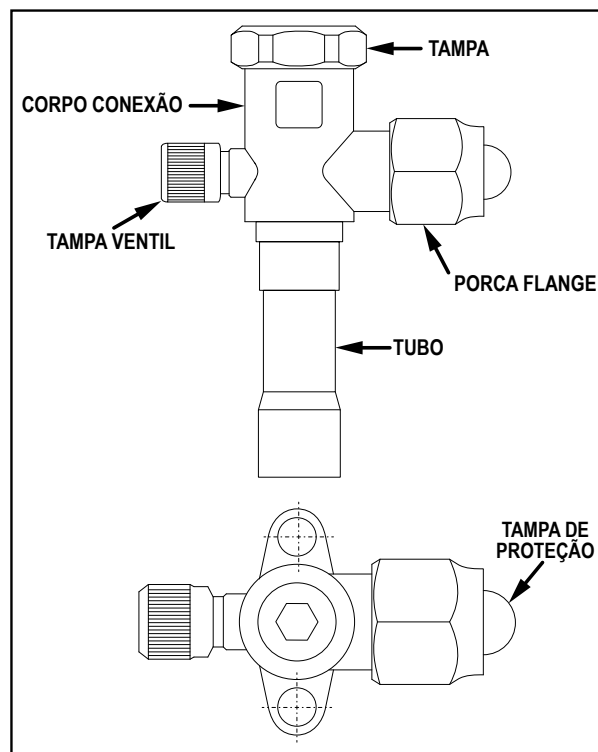
FIG. 18 - VÁLVULA DE SERVIÇO LINHAS SUÇÃO/EXPANSÃO
