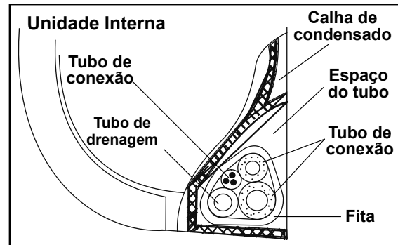
FIG. 10 - TUBO DE CONEXÕES
