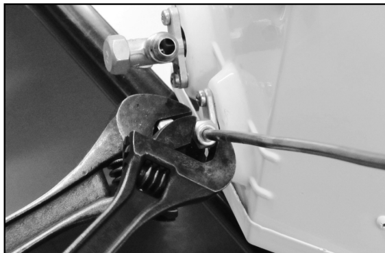
FIG. 25 - FIXAÇÃO DA PORCA
