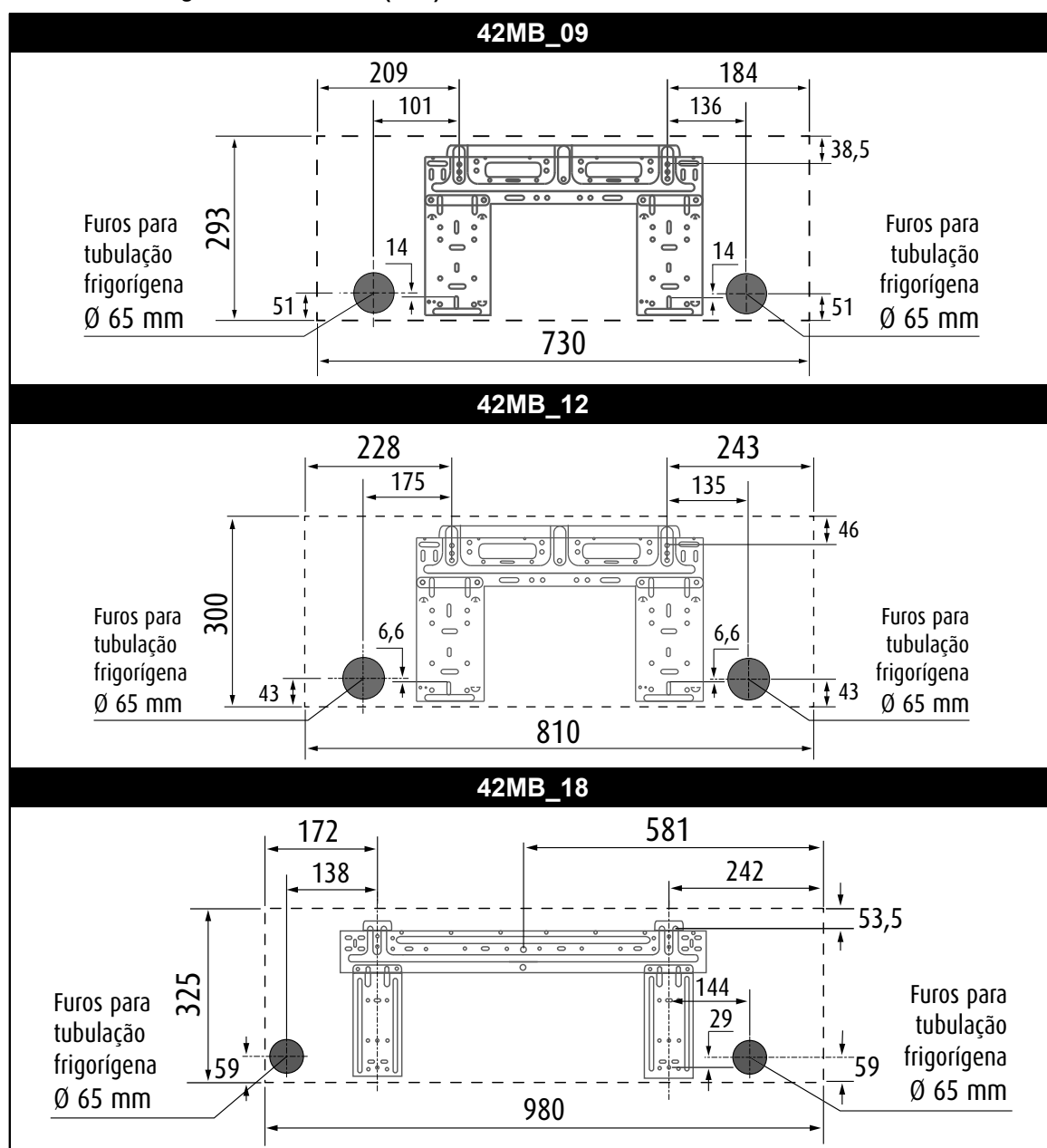
FIG. 14-A - PLACAS DE MONTAGEM
